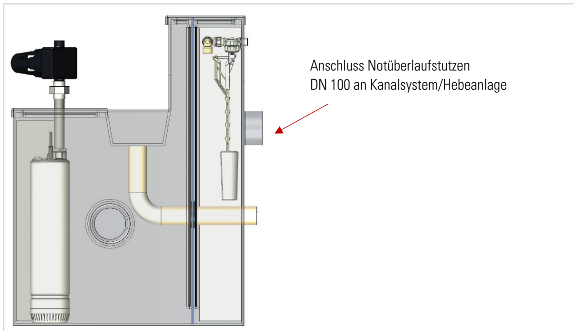
Abbildung 7: Notüberlauf Typ AB
