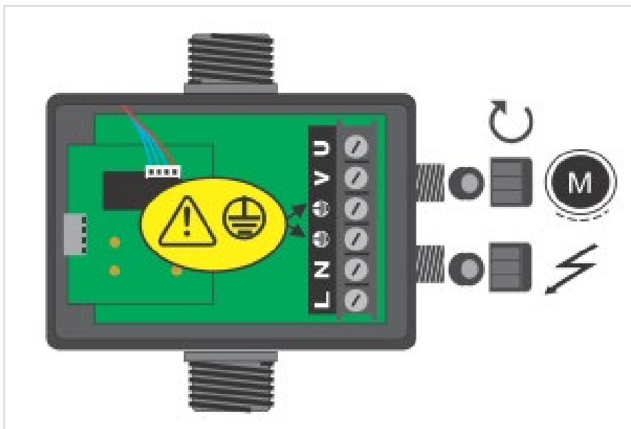
Abbildung 8: Elektrischer Anschluss
