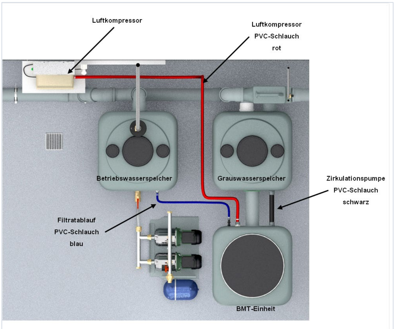
Abbildung 11: Schlauchleitungen für Belüftung, Zirkulation und Filtrat anschließen
