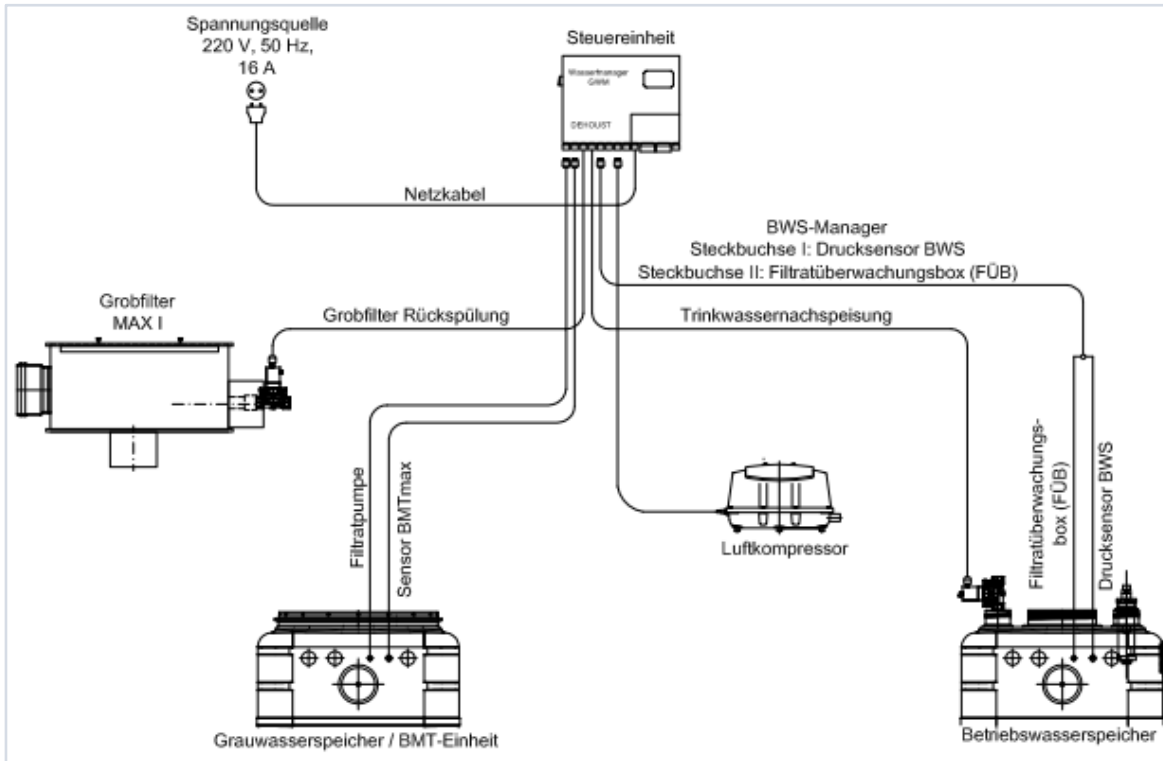
Abbildung 23: Elektrischer Anschluss von Grobfilter, Grauwasser- und Betriebspeicher GWM 500
