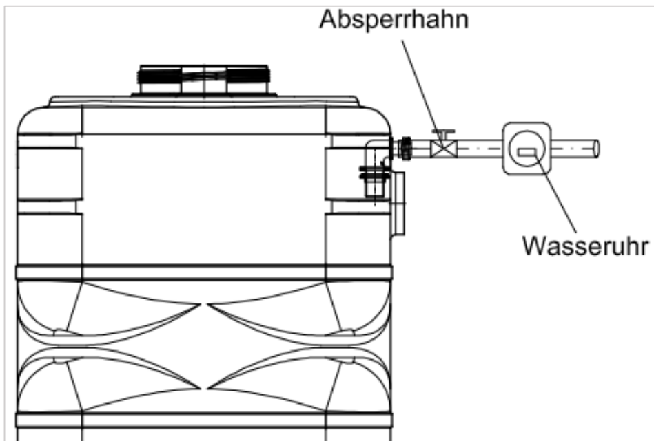
Abbildung 17: Anschluss der Betriebswasserleitung bei integrierter Tauchdruckpumpe
