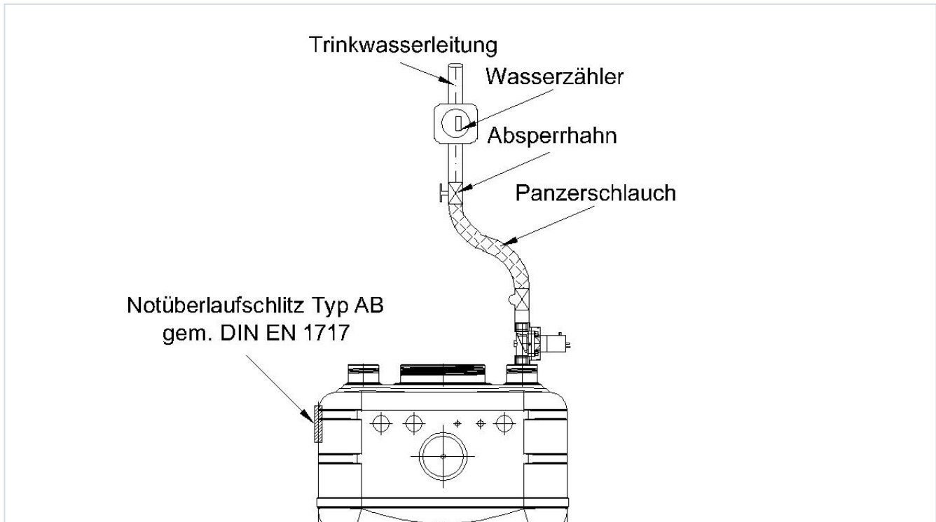
Abbildung 16: Anschluss der Trinkwassernachspeisung
