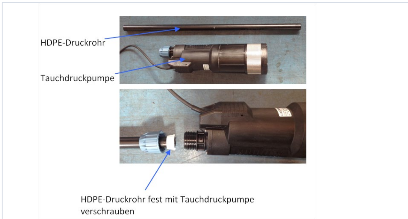
Abbildung 15: Verbindung von HDPE-Druckrohr mit Tauchdruckpumpe
