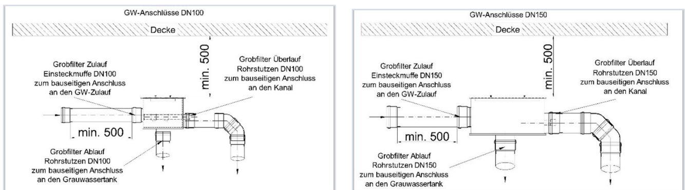
Abbildung 6: Anschluss der Rückspülung am Grobfilter DEHOUST MAX I und MAX II
