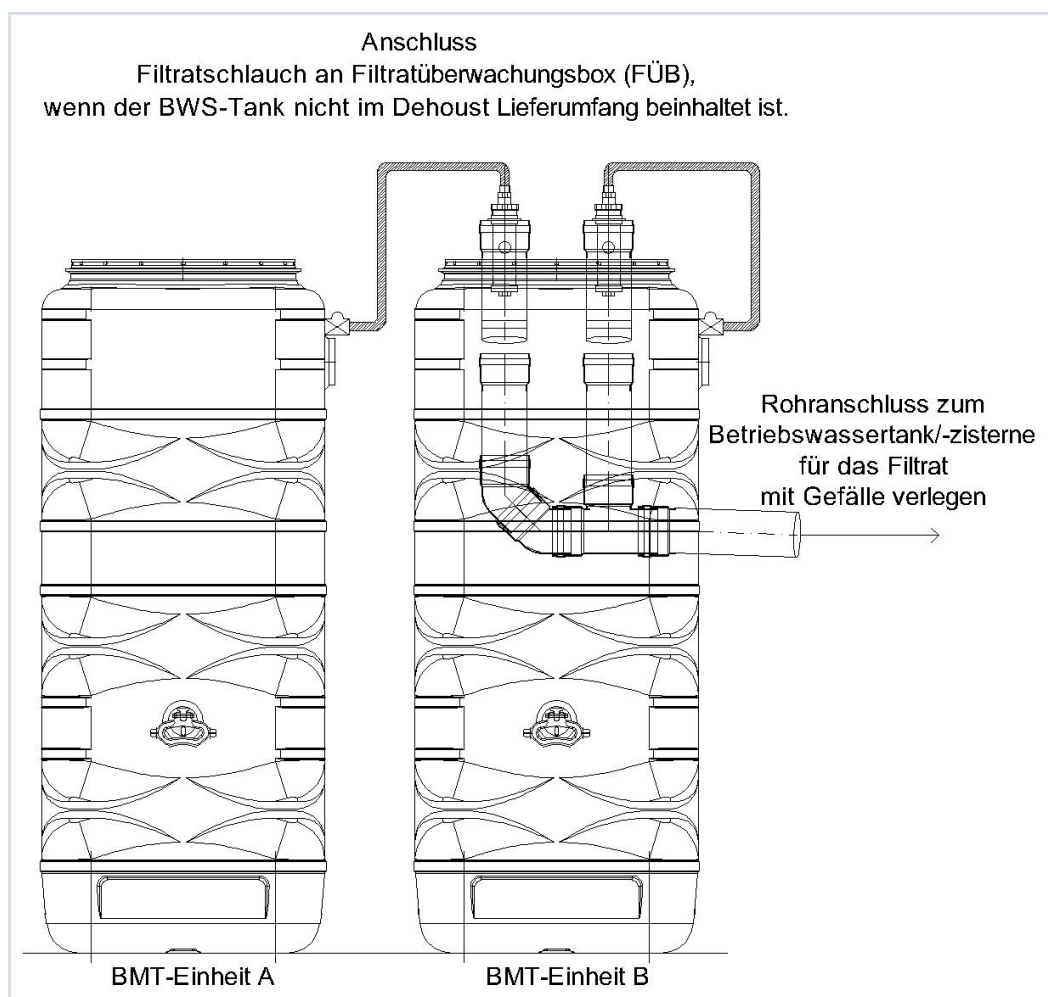
Abbildung 13: Anschluss Filtratschlauch an FÜB der BMT-Einheit bei bauseitigem Betriebswasserspeicher Variante 1
