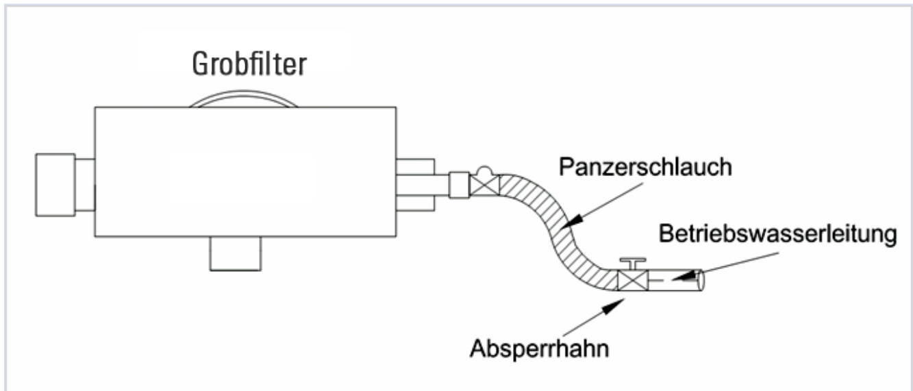
Abbildung 5: Anschluss der Rückspülung
