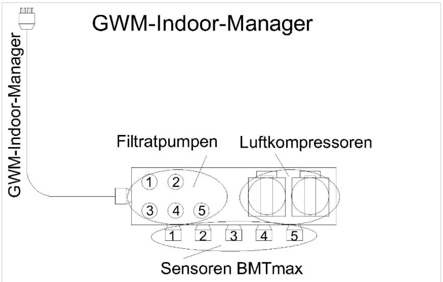
Abbildung 22: Anschlüsse auf dem GWM-Indoor-Manager
