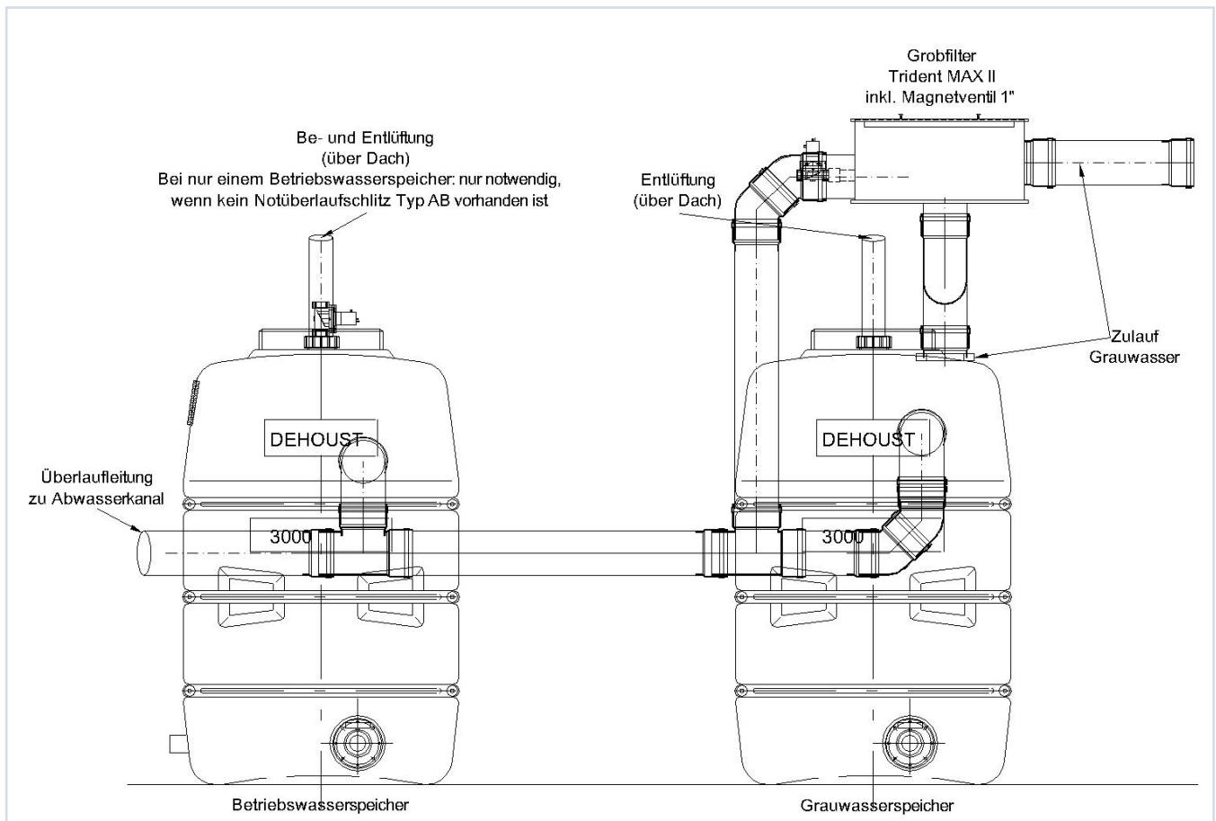
Abbildung 8: Anschluss der Überläufe an DF-Tanks
