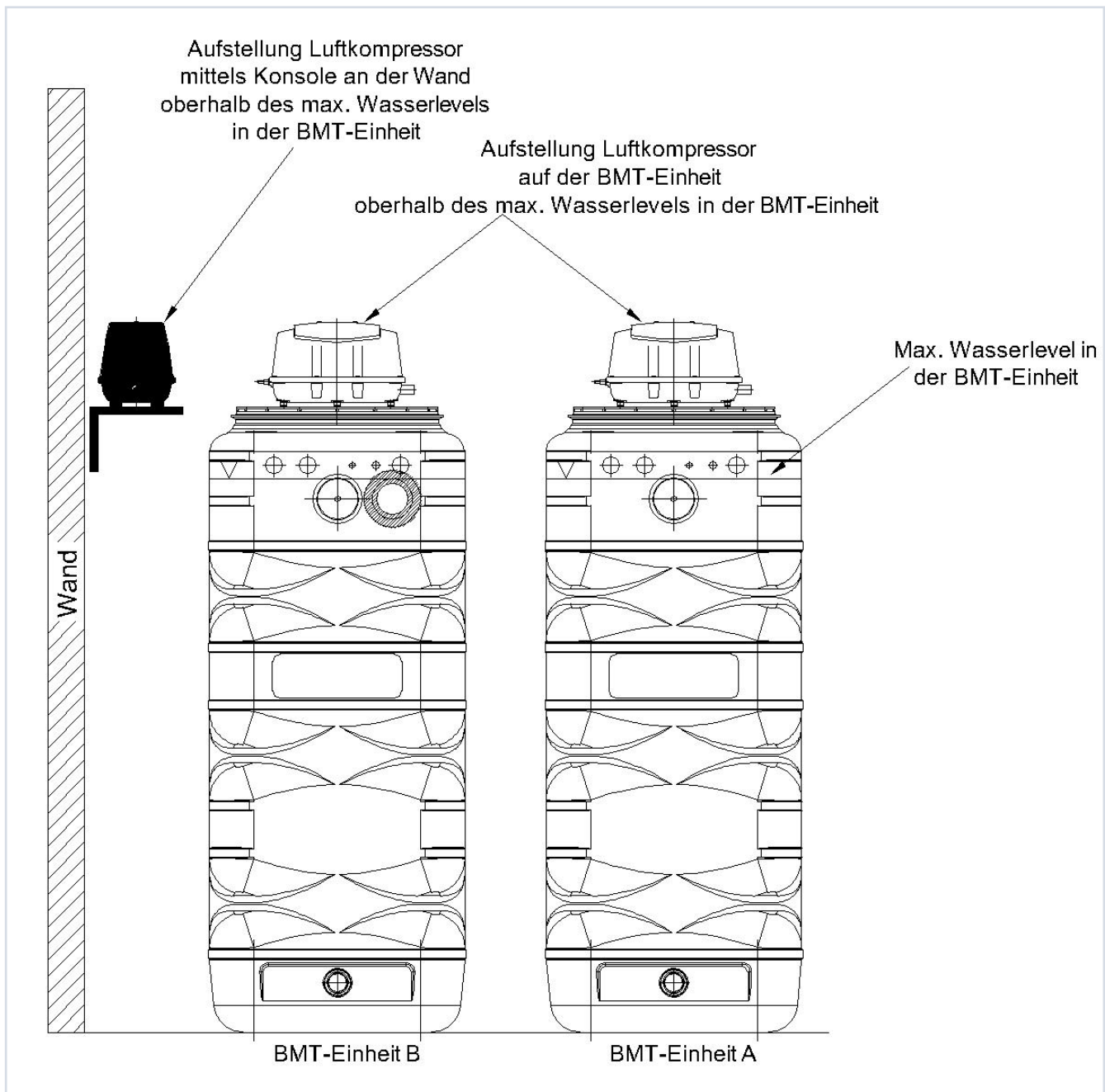
Abbildung 12: Aufstellung des Luftkompressors
