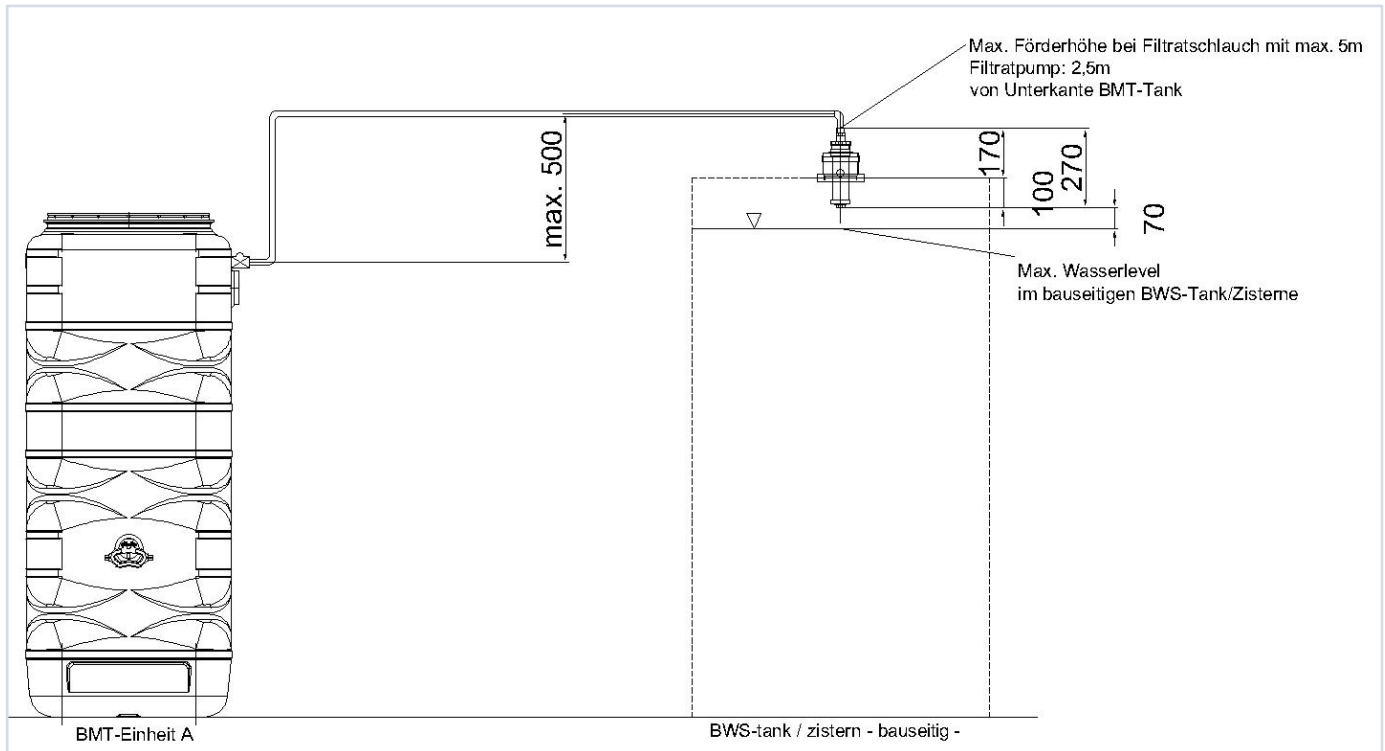
Abbildung 14: Anschluss Filtratschlauch an FÜB der BMT-Einheit bei bauseitigem Betriebswasserspeicher Variante 2
