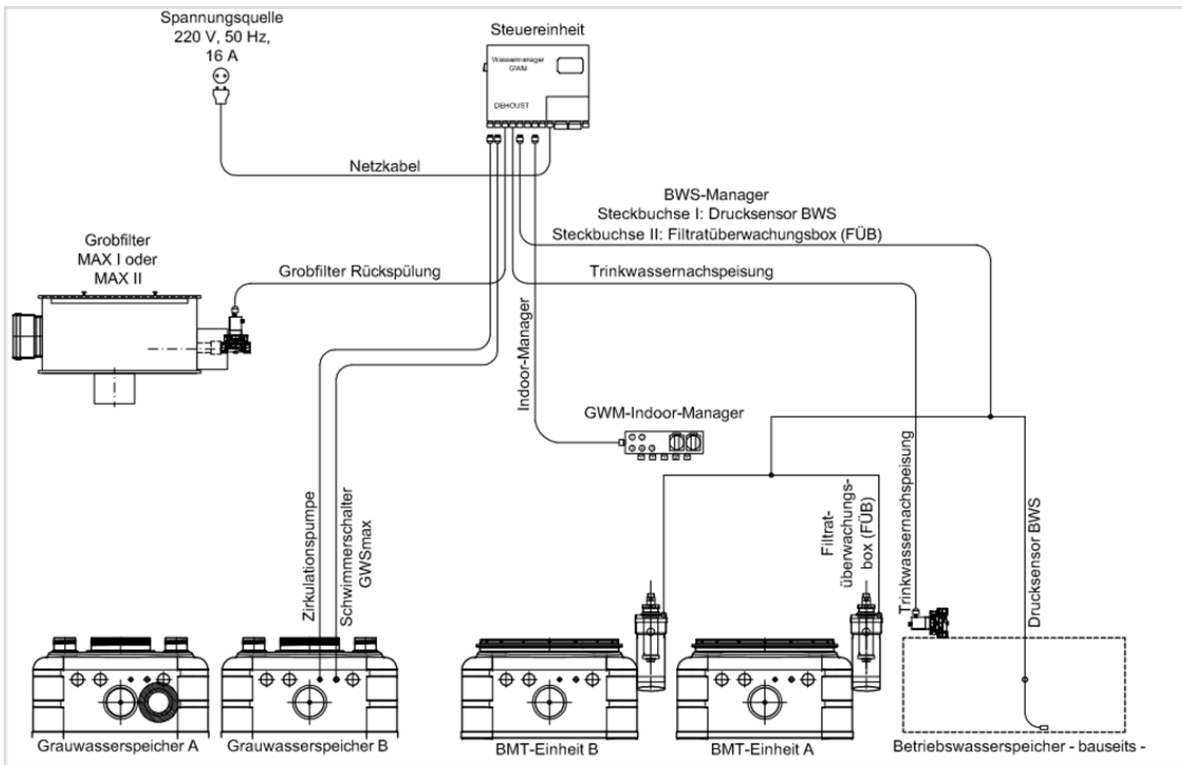
Abbildung 25: Elektrischer Anschluss von Grobfilter, Grauwasser- und bauseitigem Betriebswasserspeicher GWM 950 (Variante 1)
