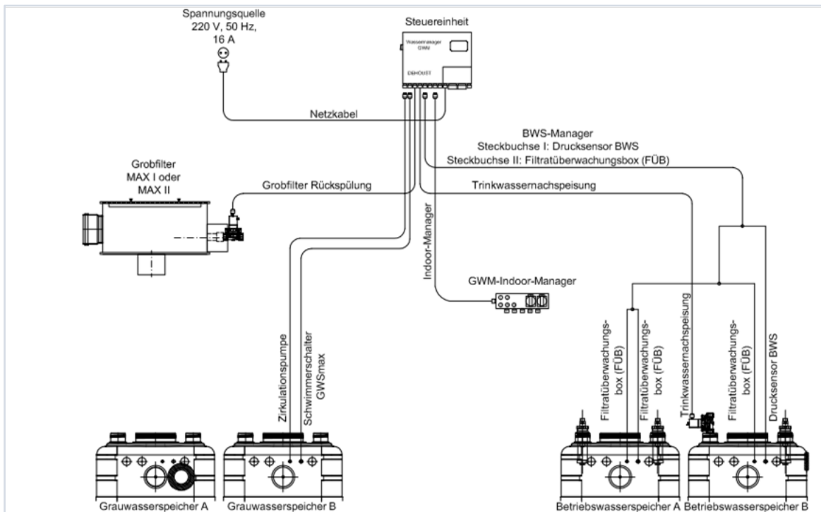
Abbildung 24: Elektrischer Anschluss von Grobfilter, Grauwasser- und Betriebspeicher GWM 950+
