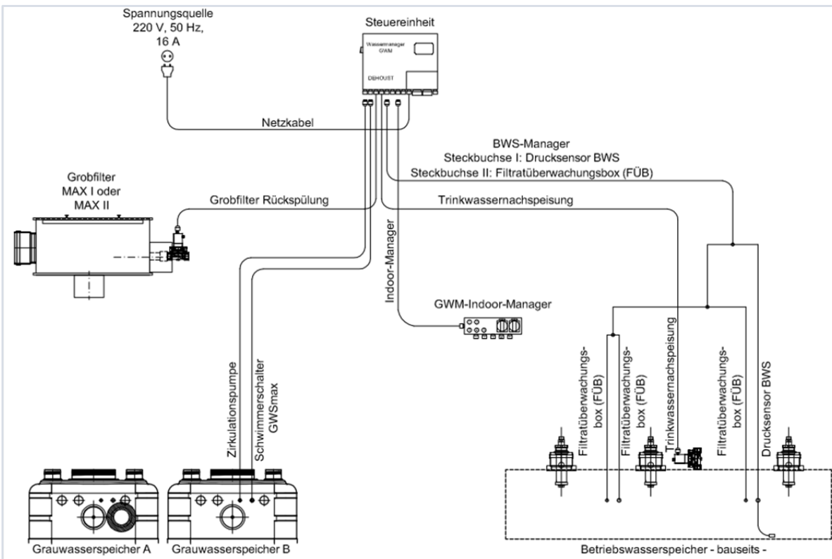
Abbildung 26: Elektrischer Anschluss von Grobfilter, Grauwasser- und bauseitigem Betriebswasserspeicher GWM 950+ (Variante 2)
