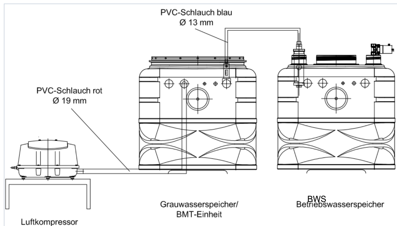
Abbildung 10: Schlauchleitungen für Belüftung und Filtrat anschließen
