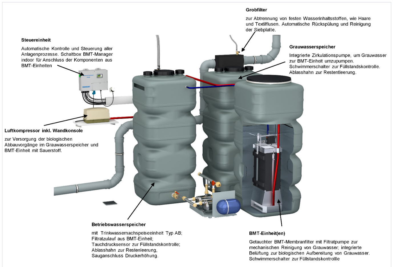
Abbildung 1: prinzipieller Aufbau des Wassermanagers
