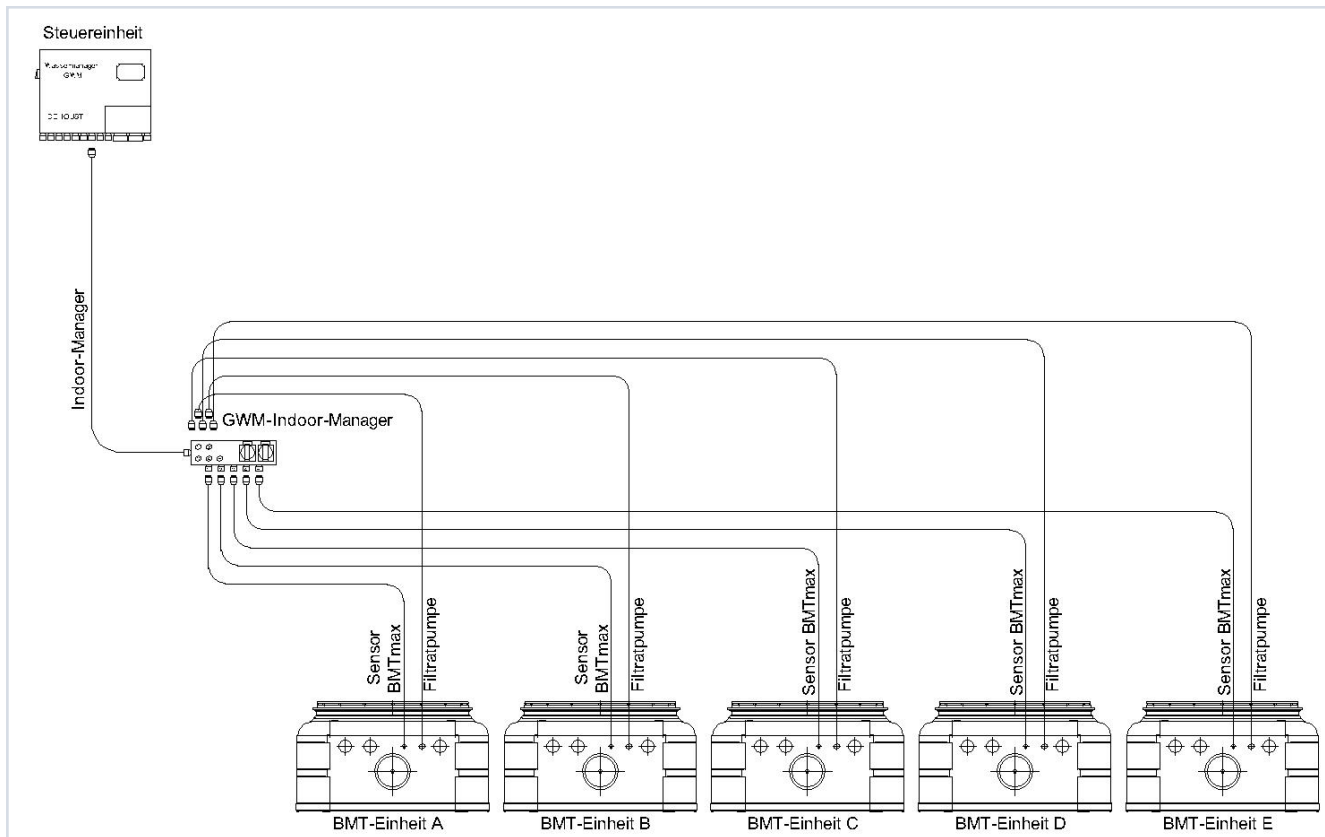
Abbildung 27: Elektrischer Anschluss des GWM-Indoor-Managers mit Filtratpumpen und Sensor-BMT für GWM 950+
