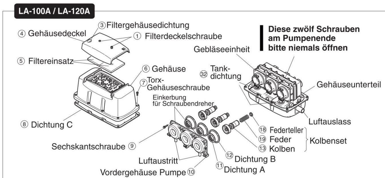
Abbildung 34: Explosionszeichnung Luftfilter Luftkompressor
