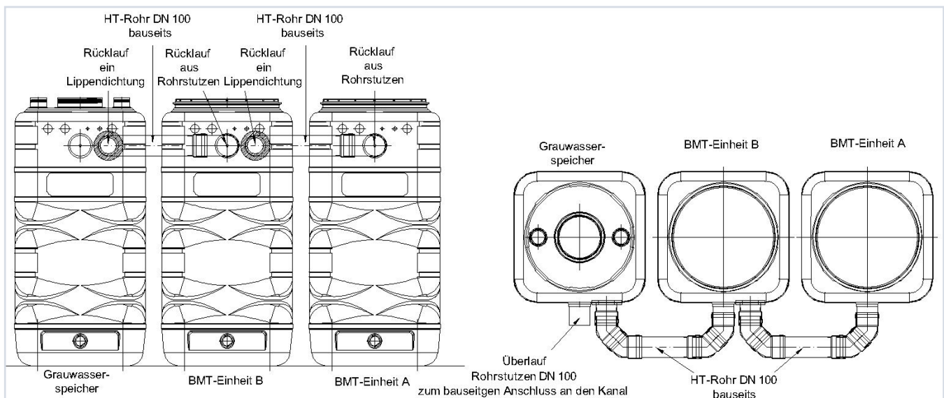
Abbildung 9: Anschluss des Grauwasserrücklaufs
