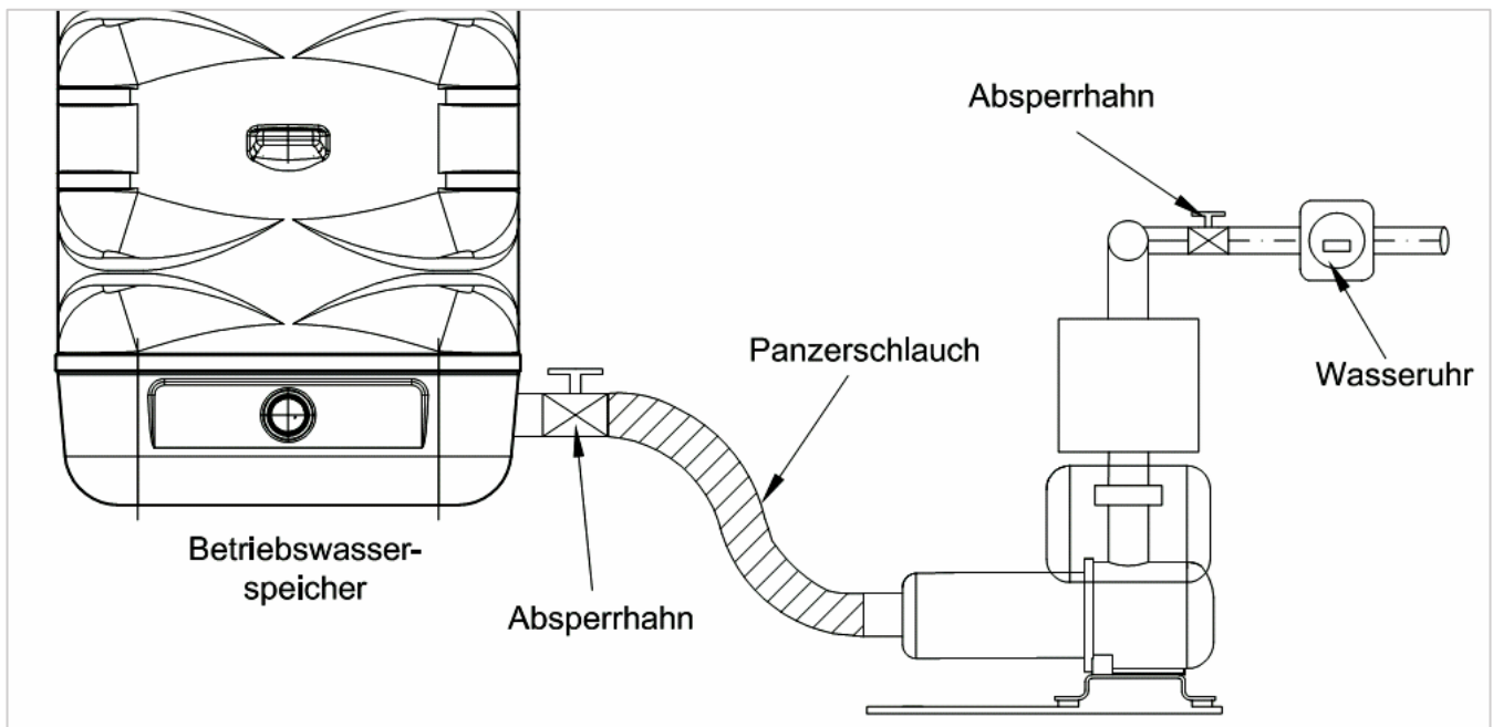
Abbildung 19: Anschluss der Betriebswasserleitung mit trocken aufgestellter Druckerhöhungsanlage bei GWM 500
