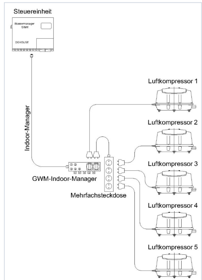
Abbildung 29: Anschluss von bis zu fünf Luftkompressoren am GWM-Indoor-Manager
