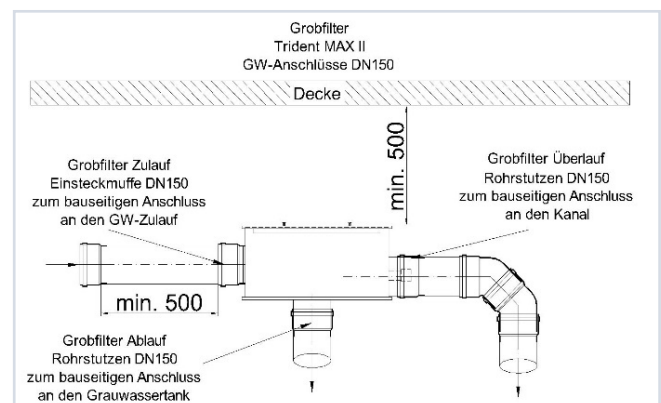
Abbildung 4: Anschluss des Grobfilters MAX II
