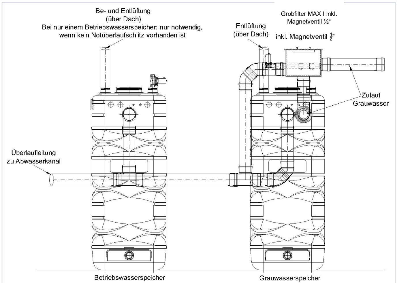
Abbildung 7: Anschluss der Überläufe an AQF-Tanks
