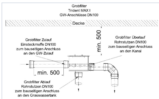
Abbildung 3: Anschluss des Grobfilters MAX I
