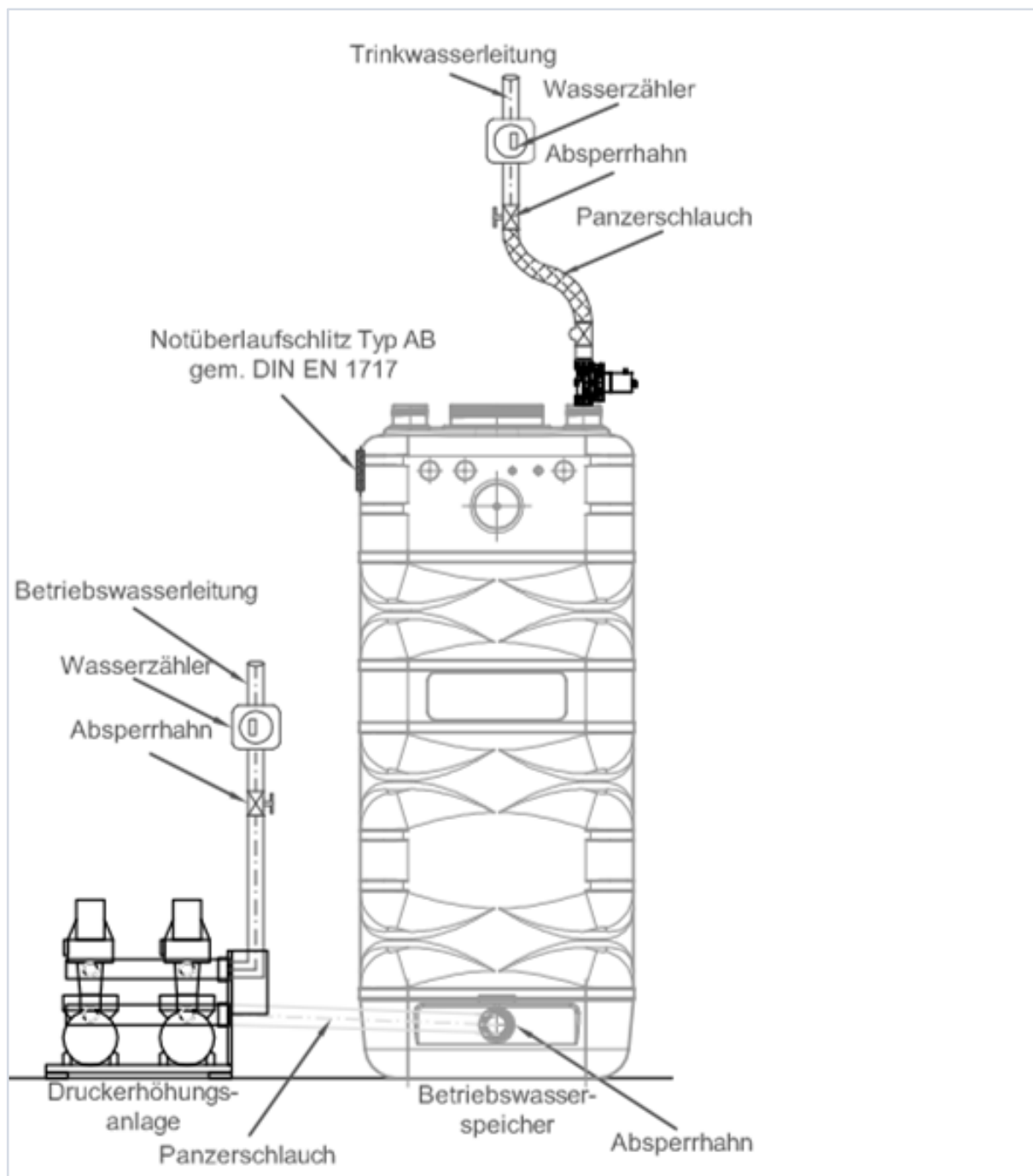
Abbildung 18: Anschluss der Betriebswasserleitung bei GWM 950+
