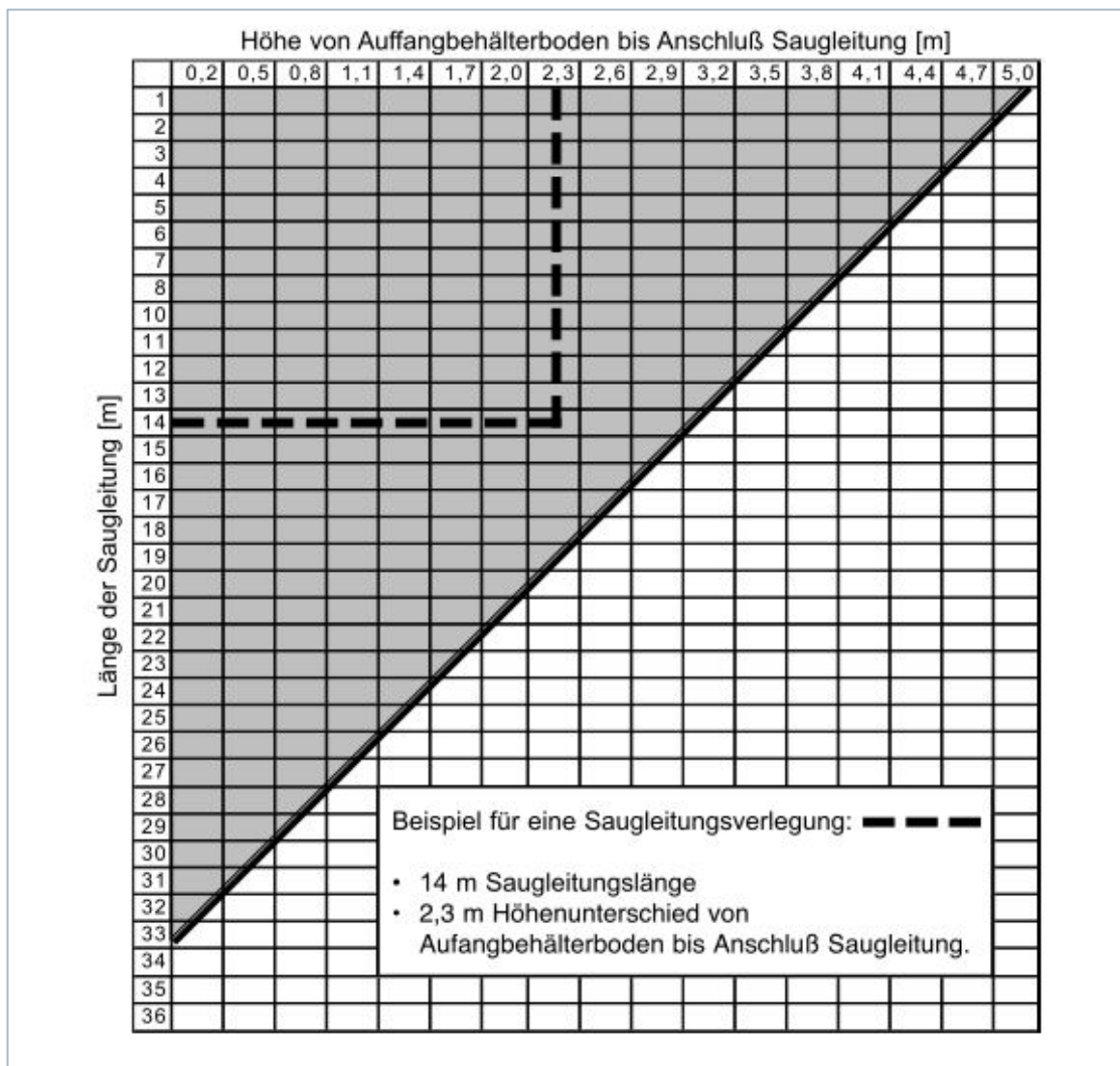
Abbildung 6: Darstellung Verhältnis Länge der Saugleitung zu Höhe vom Auffangbehälterboden (z. B. Zisterne/ Erdbehälter) bis Anschluss-Saugleitung; Bemessungsgrundlage der Tabelle: 1"PE-Saugleitung (25 mm Innendurchmesser) bei einem verbraucherbedingten Spitzendurchfluss von max. 3 m³/h.
