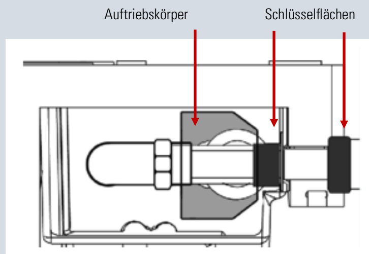
Abbildung 5: Trinkwassernachspeisung Innenansicht
