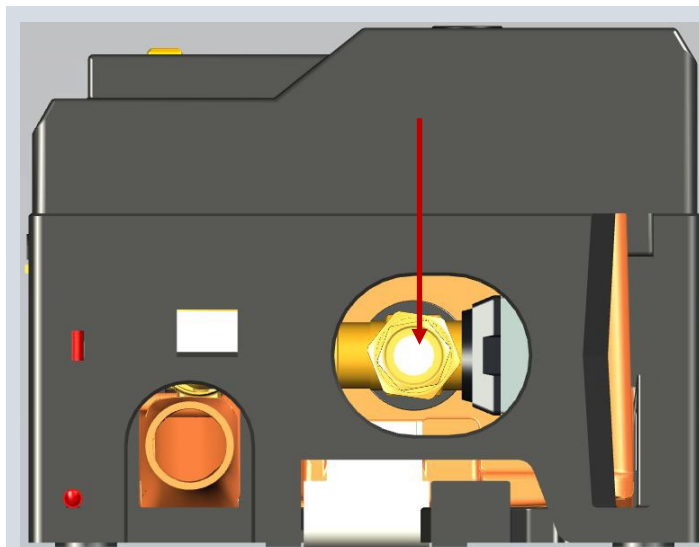
Abbildung 7: Der Sauganschluss (Ansicht von unten)
