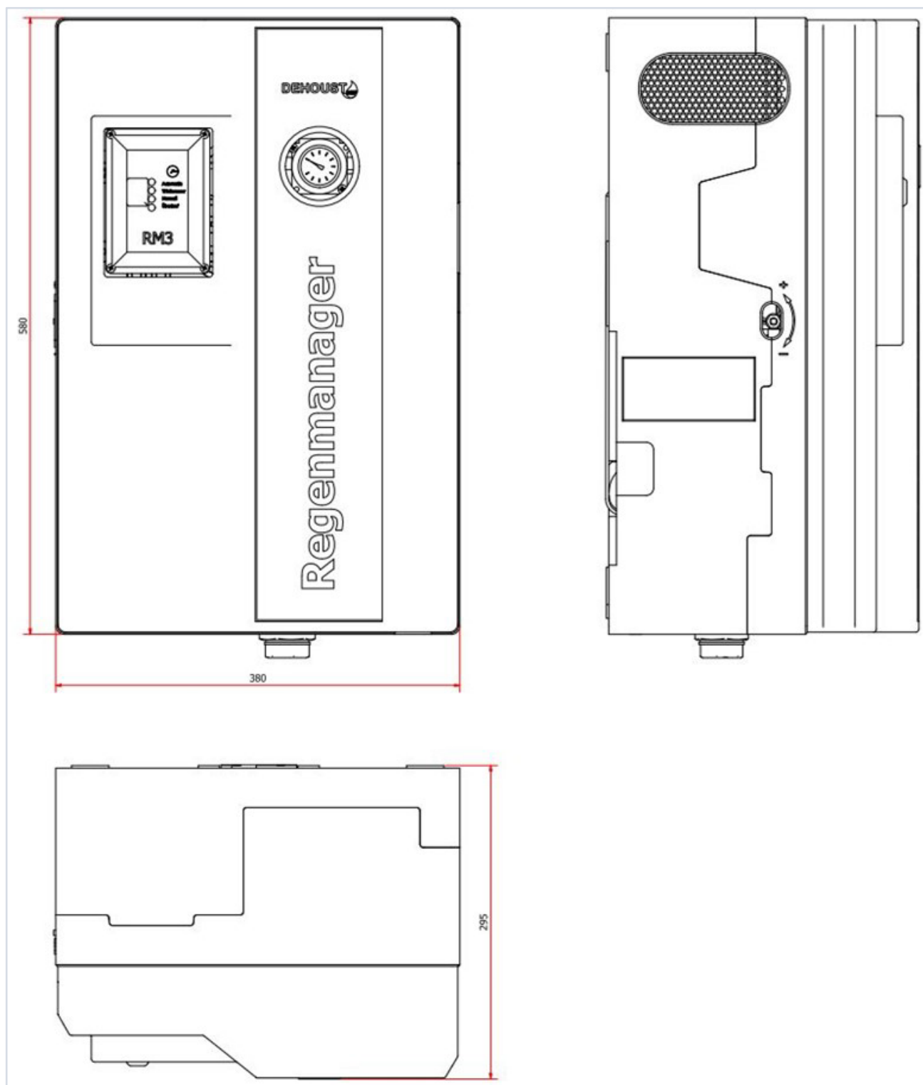
Abbildung 2: Außenmaße
