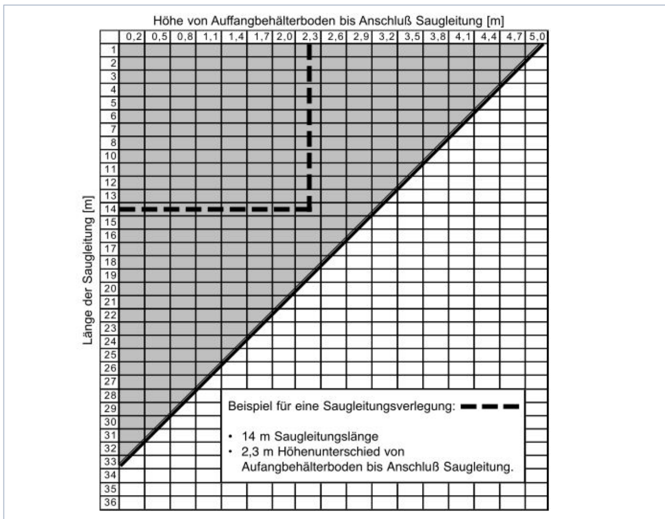
Abbildung 7: Darstellung Verhältnis Länge der Saugleitung zu Höhe vom Auffangbehälterboden (z. B. Zisterne/ Erdbehälter) bis Anschluss-Saugleitung; Bemessungsgrundlage der Tabelle: 1"PE-Saugleitung (25 mm Innendurchmesser) bei einem verbraucherbedingten Spitzendurchfluss von max. 5 m³/h.
