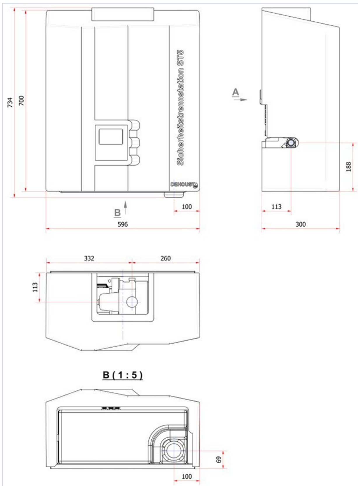
Abbildung 2: Außenmaße
