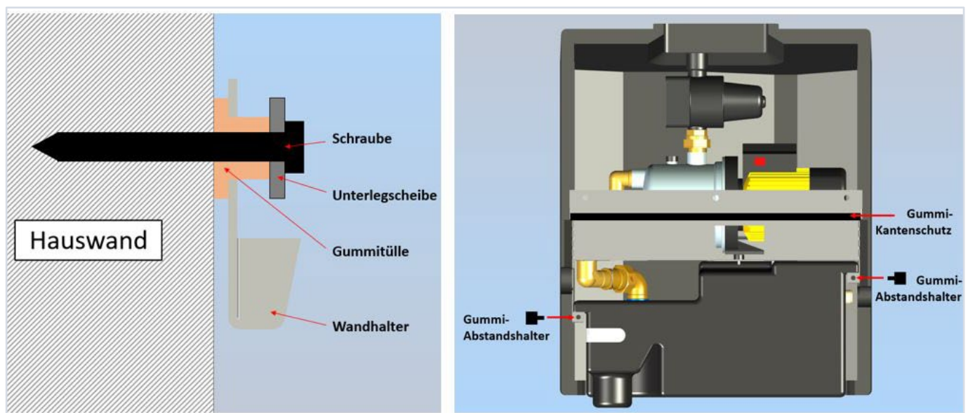
Abbildung 4: Wandmontage der Sicherheitstrennstation ST 5-3,2 - Bild links / Bild rechts
